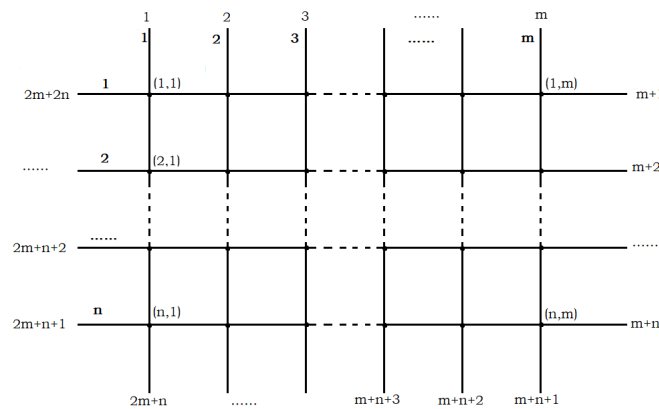
图 2: 射线的编号
